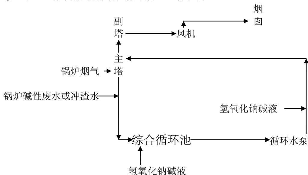
民丰特纸热电蒸汽锅炉烟气脱硫除尘系统污染治理工艺示意图 ①#9 和#10 链条蒸汽锅炉烟气脱硫除尘一体化装置：
